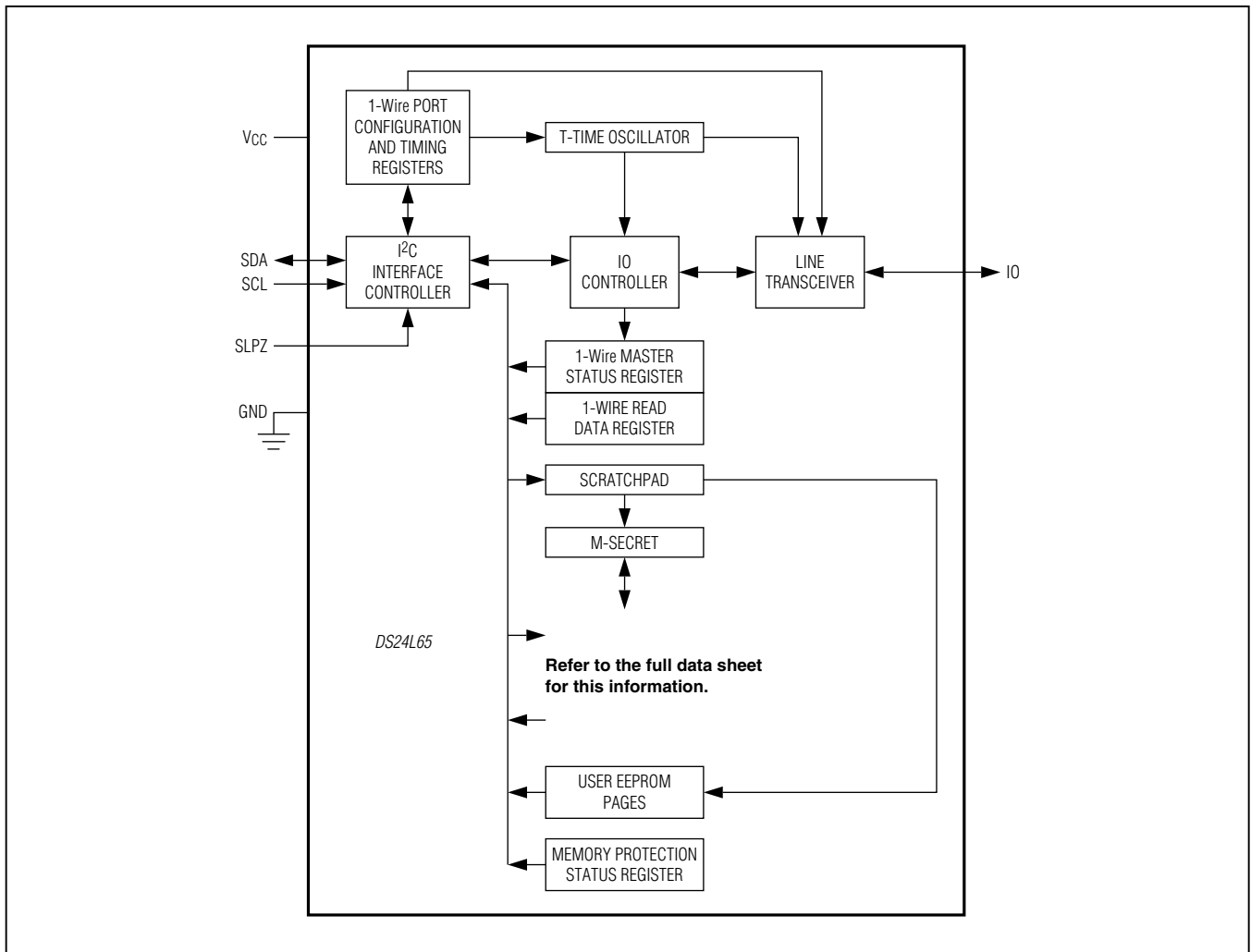
图1. 方框图
