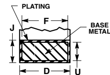
VIEW Y
